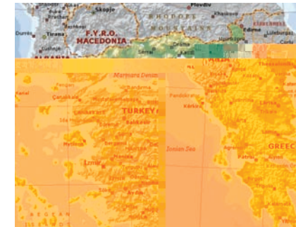
[그림 2-5] 그리스 섬 분포와 산토리니 섬
