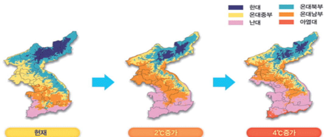
:그림 IV+20< 기온상승에 따른 한반도 기후변화
