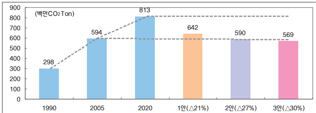
<그림 IV-39> 온실가스 배출량 추이 및 감축 시나리오
