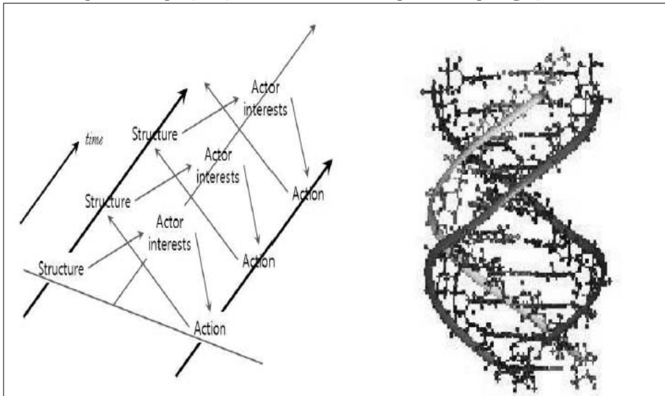
[그림 2-4] 네트워크모델
