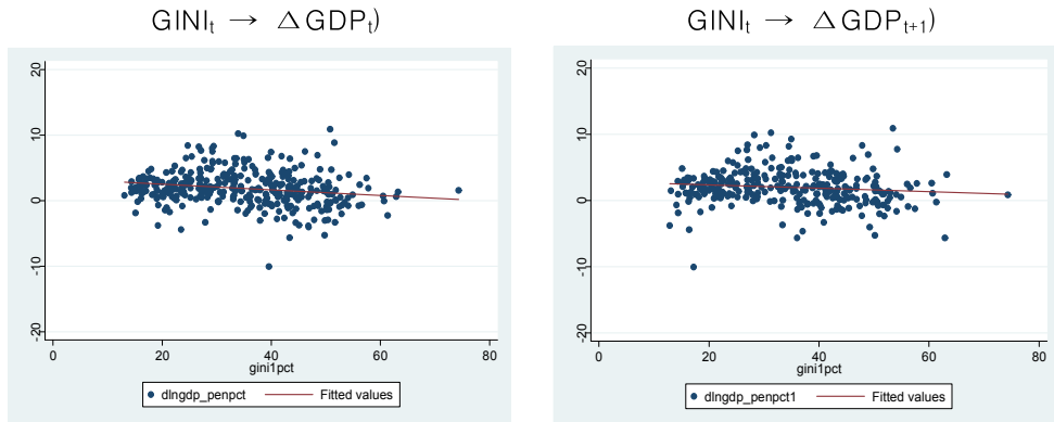
<그림 IV-1> 소득불균등 정도 X )와 경제성장률 Y )의 산포도
