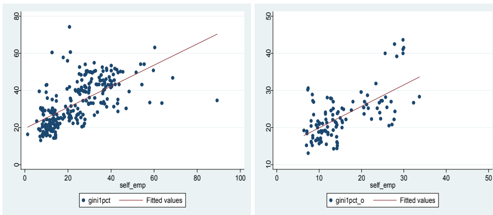
<그림 III-8> 자영업자비중 X )과 소득불균등정도 Y ) 간 산포도 전체 국가) OECD 국가)
