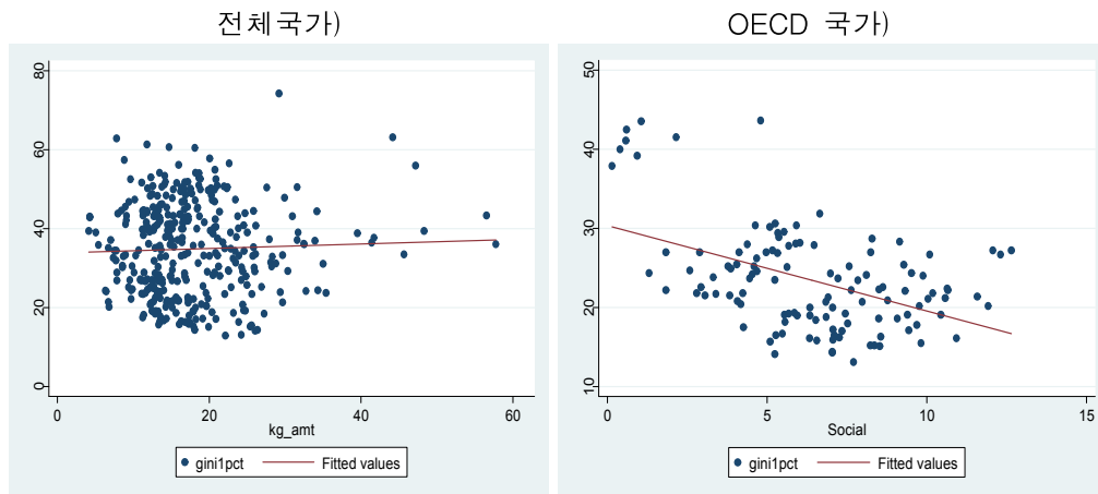
<그림 III-6> 정부지출비중 X )과 소득불균등정도 Y ) 간 산포도
