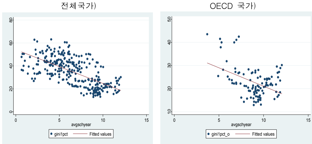
<그림 III-4> 평균 교육년수 X )와 소득불균등정도 Y ) 간 산포도
