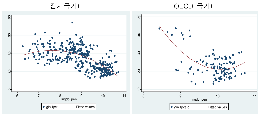
<그림 III-3> 일인당 소득수준 X )과 소득불균등정도 Y ) 간 산포도
