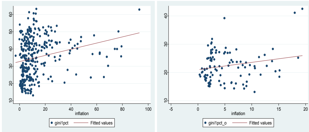
<그림 III-9> 인플레이션율 X )과 소득불균등정도 Y ) 간 산포도 전체 국가) OECD 국가)
