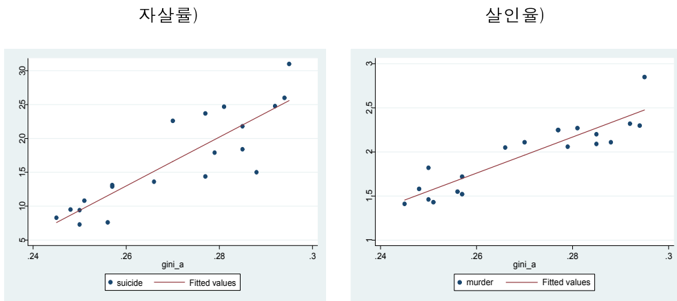
<그림 III-1> 우리나라 소득불균등 X )과 자살률 및 범죄율 Y )간 산포도
