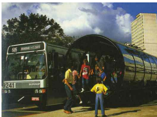
〈그림 3-12〉 원통형 버스정류장
