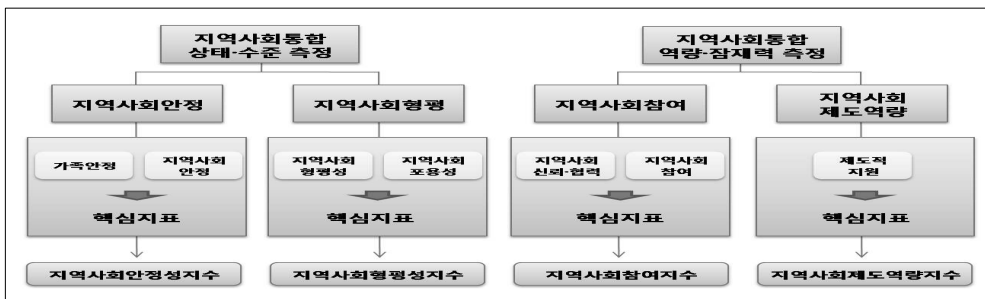
그림 7-1 지역사회통합지수 산출구조
