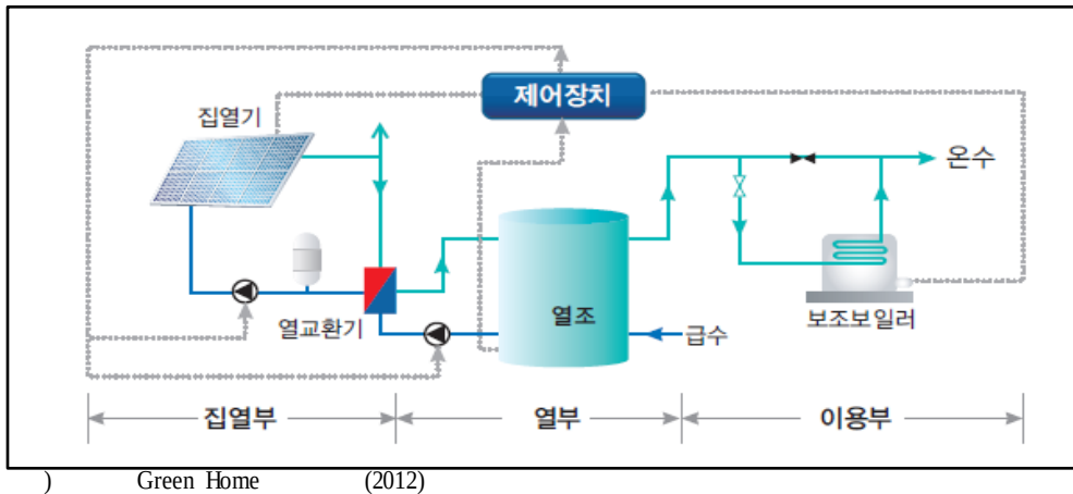
(그림8) 태양열 시스템 구성도
