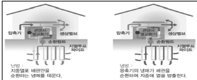
(그림9) 지열시스템 구성도
