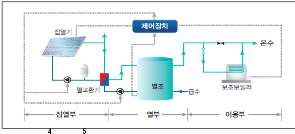
(그림8) 태양열 시스템 구성도
