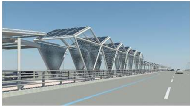
<그 16> 중 분리대 태양 설치모형(하단부는 자전거도로)
